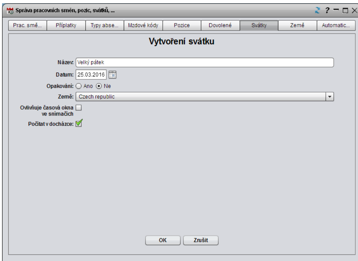
Obr. 3 – Dialogové okno pro vytvoření nového svátku
